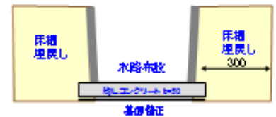
水路工 標準断面図
